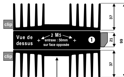
2 radiateurs additifs pour modèles ② et ③
